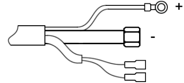
Раздельное подключение
